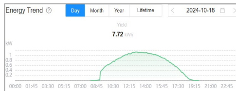
Curva de producción día medio
